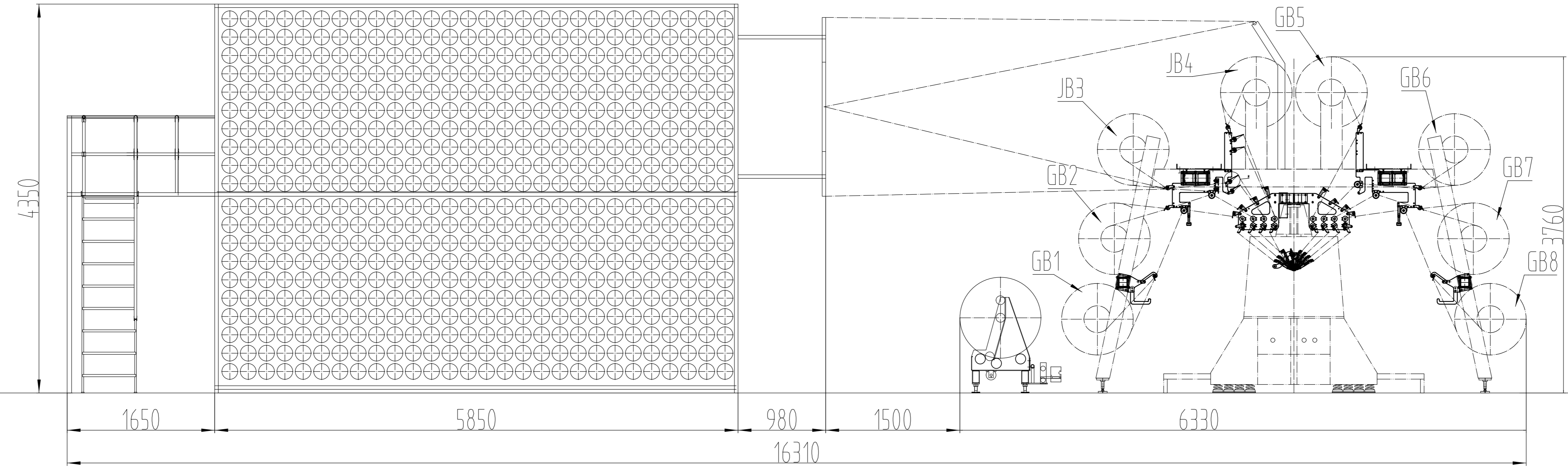
3360纱架+料台
